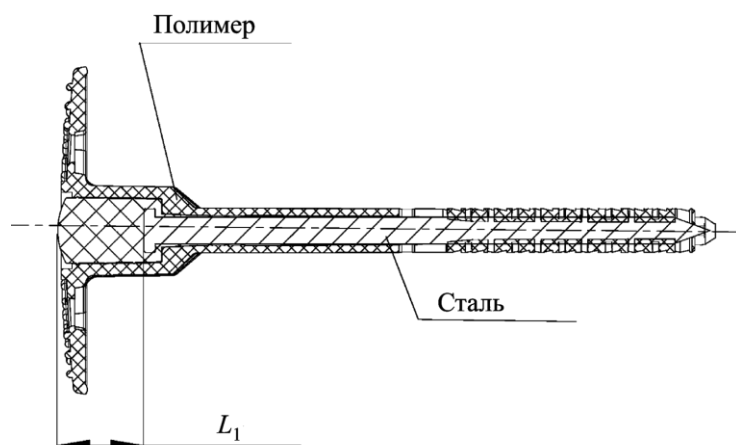
Рисунок Г.2 – Схема тарельчатого анкера
