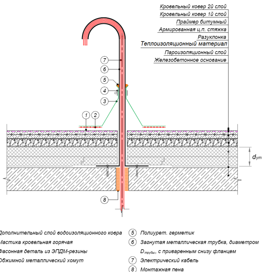
Рисунок Г.10 – Схема пропуски электрического кабеля через совмещенное кровельное покрытие
